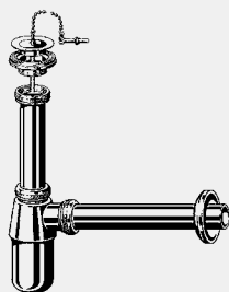
Сифон тип бутилка Компоненти Декоративна розетка Ø 50 мм, универсален клапан от неръждаема стомана, тапа за клапан с верига Модел 5753.906
