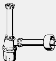
Сифон тип бутилка - Пластмаса Компоненти Удължена регулираща се вертикална тръба Модел 5725.911
